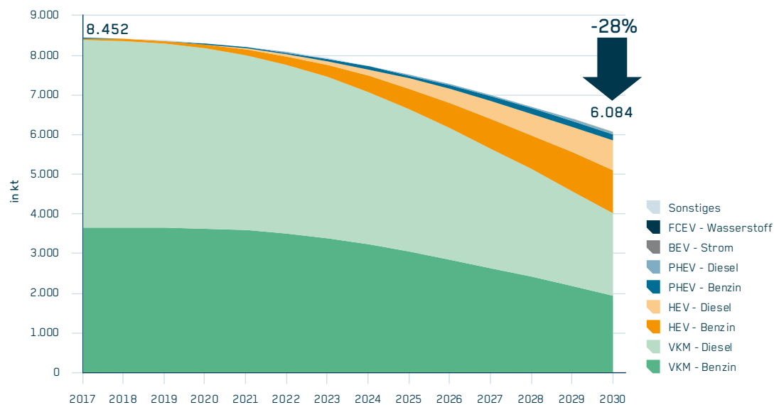
Abbildung 32: Pkw-CO 2 -Emissionen nach Technologie, Szenario 1
