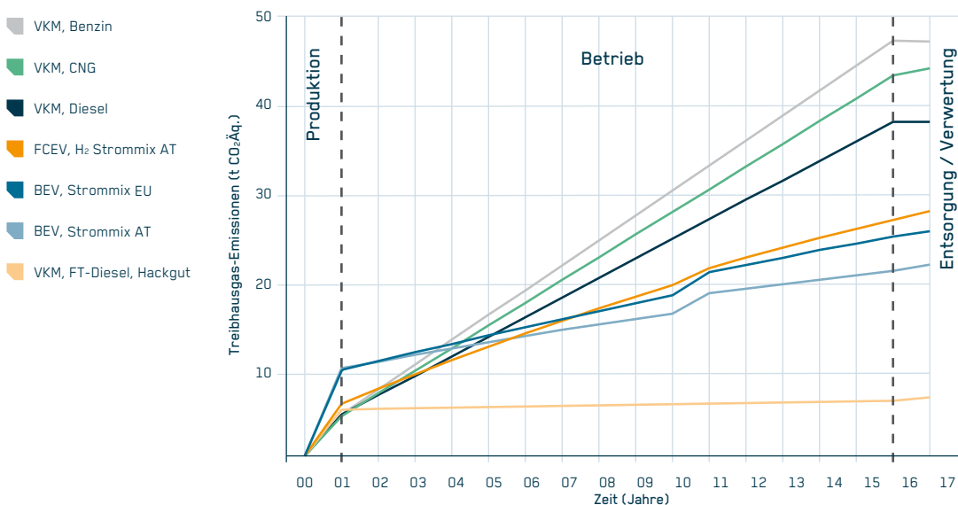
Abbildung 39: THG-Bilanz ausgewählter Antriebe im Lebenszyklus (IST-Szenario)
